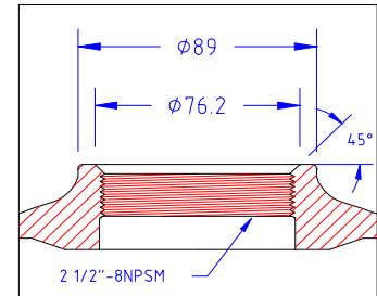
DÉTAIL FILET DE 2 1/2"
